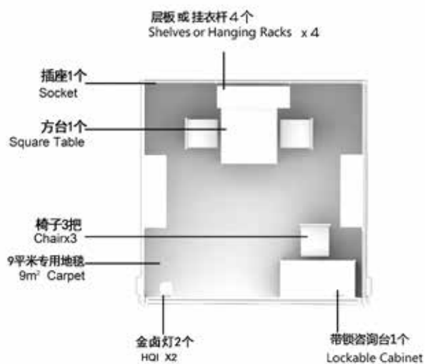
平面图
